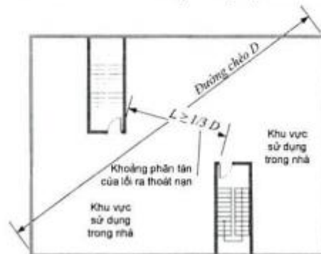
d) Trường hợp toàn nhà được bảo vệ bằng hệ thống sprinkler, có thể giảm khoảng phân tán của lối ra thoát nạn L \geq \frac{1}{3} D
