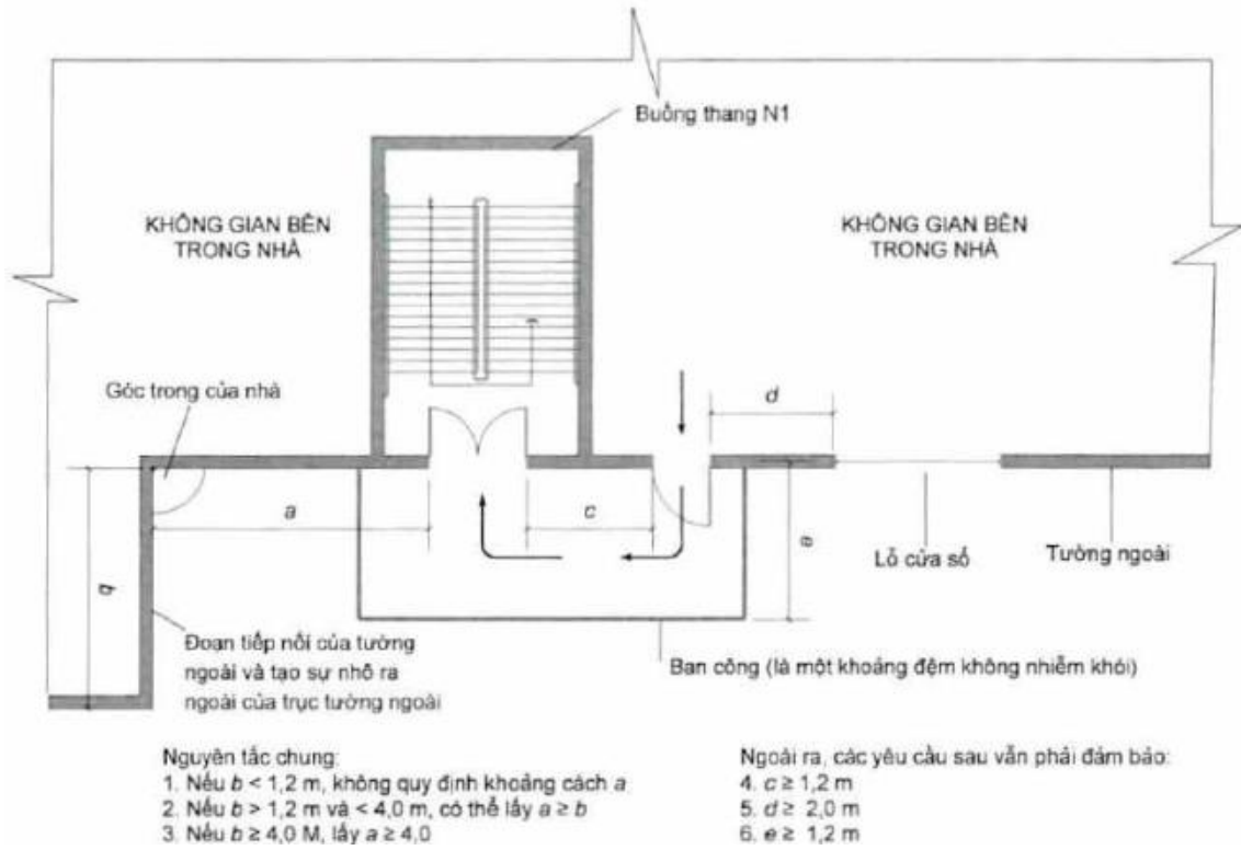
Hình I.7 - Bố trí buồng thang bộ loại N1 (xem 3.4.10 a)
