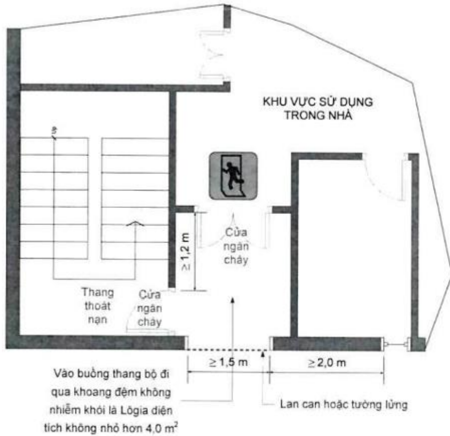
Hình I.8 - Khoảng đệm không nhiễm khói dẫn vào buồng thang bộ loại N1
